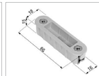
Alutop XT megfordítható zárólemez fém tokhoz
